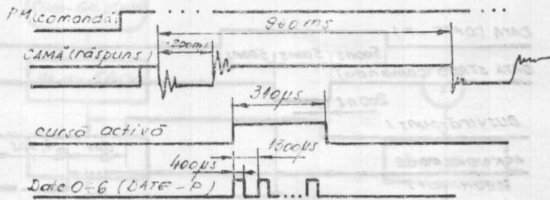
Fig. 2.2.1. Semnale dialog MIM-40.
