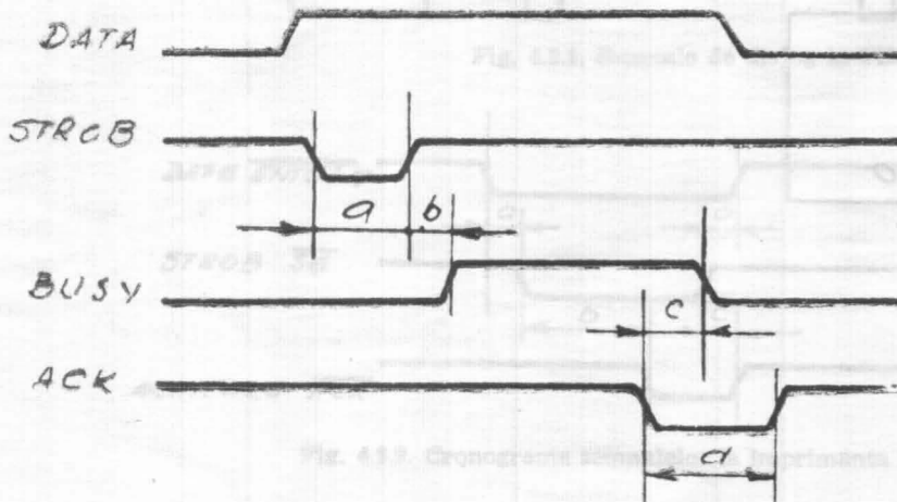
Fig. 7.2.2. Cronograma semnalelor pentru interfața paralelă.
